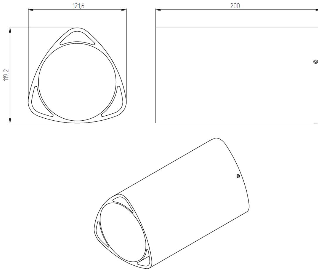
Рисунок 1. Общий вид светильника TETRA TOP 18
