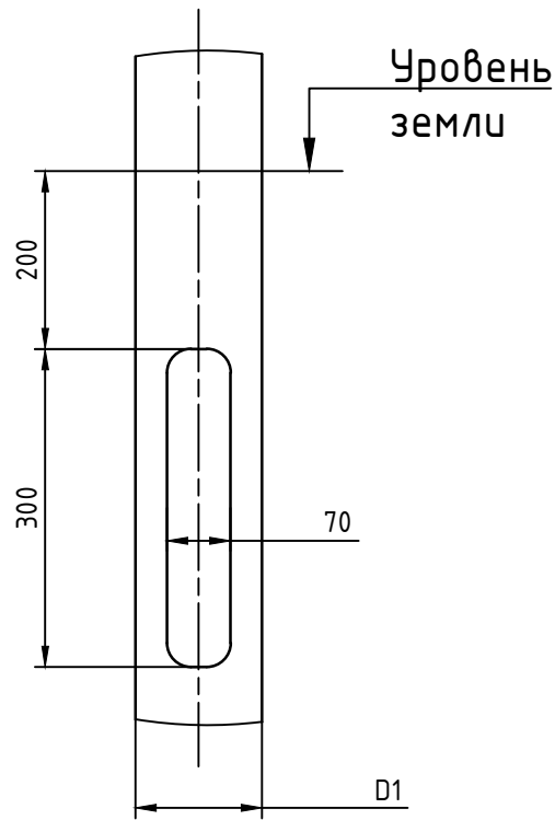
Вид В
