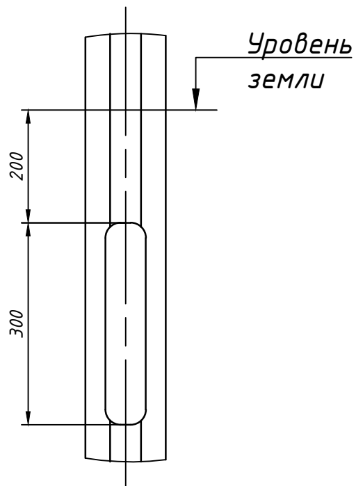
Вид В
