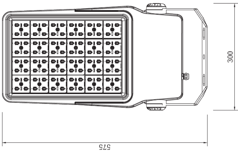
Рисунок 3. Общий вид светильника RAD-COMBO
