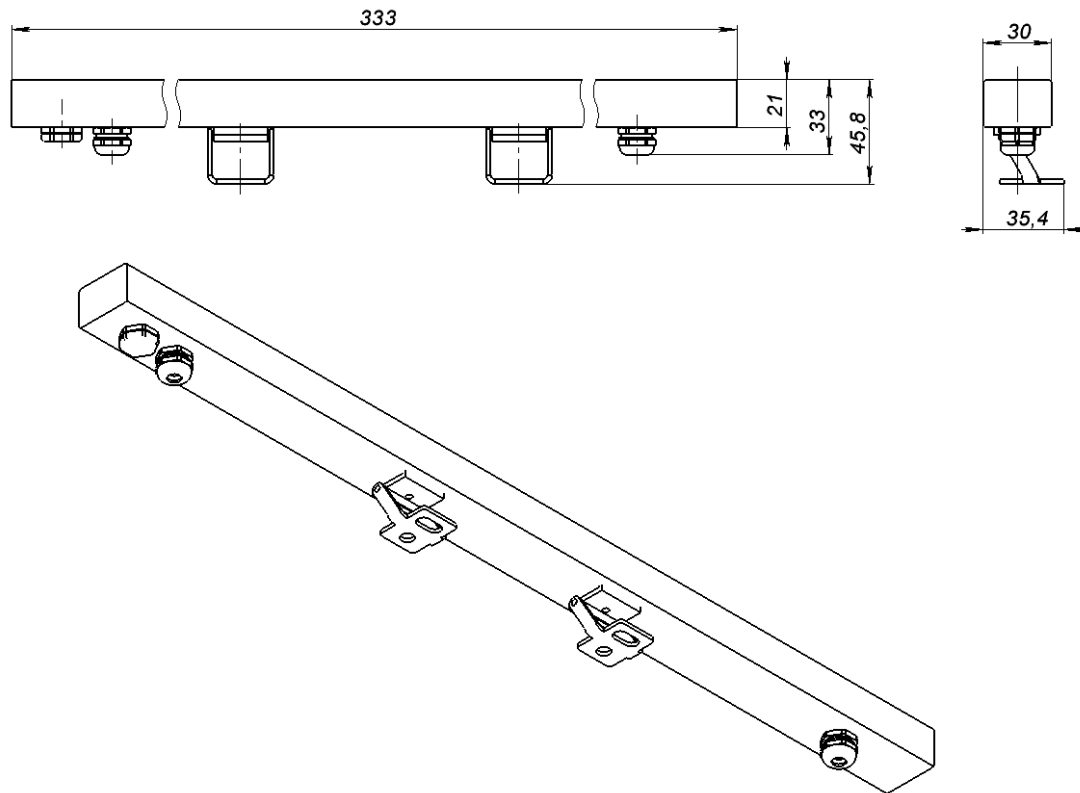
Рисунок 1. Общий вид светильника RAD-L-SL
