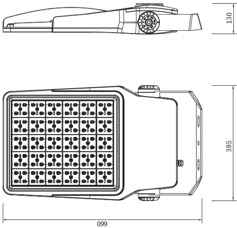
Рисунок 3. Общий вид светильника RAD-COMBO XL
