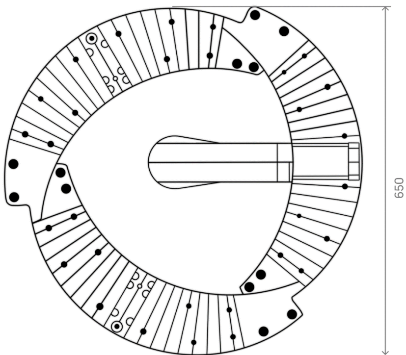
Рисунок 3. Общий вид светильника RAD-NIMB Z
