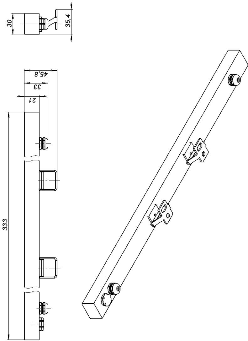
Рисунок 1. Общий вид светильника RAD-L-SL
