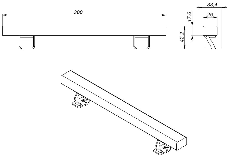
Рисунок 1. Общий вид светильника RAD-L-Mu
