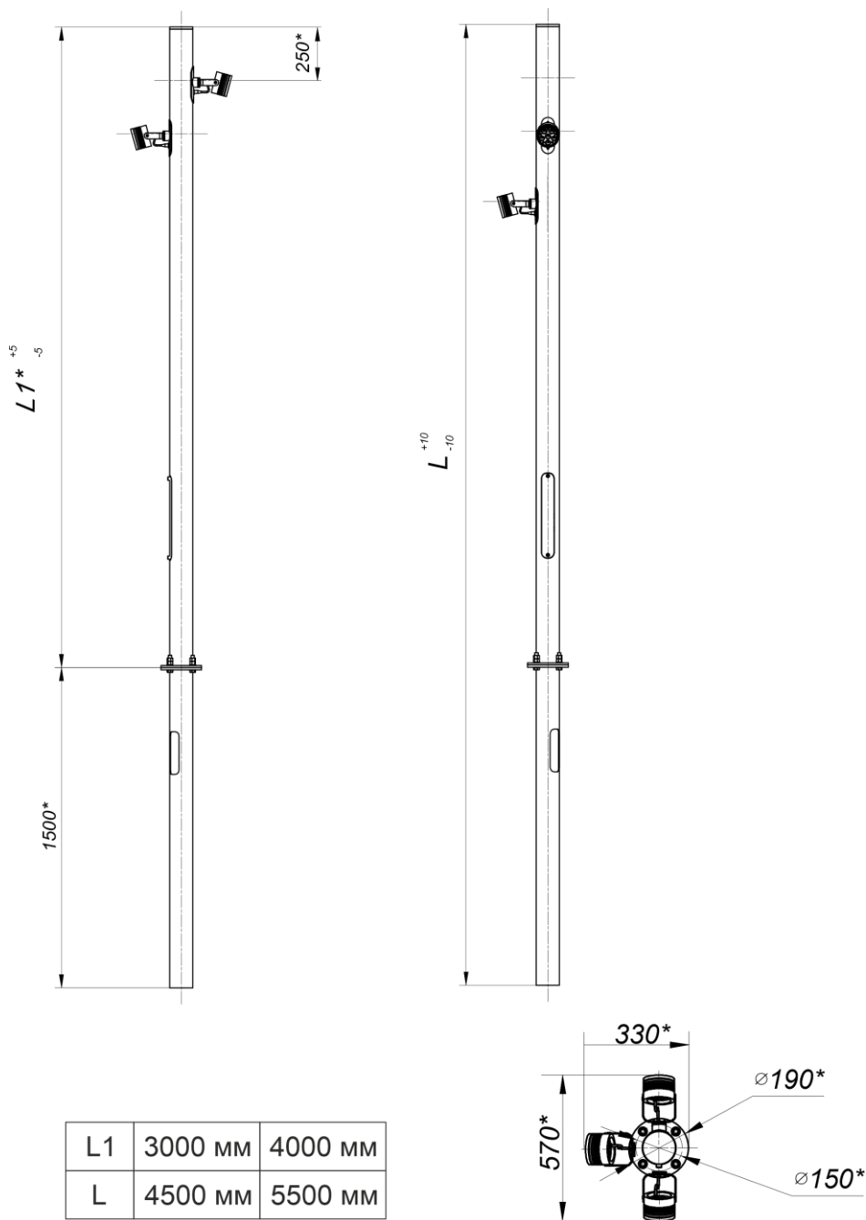
Рисунок 3. Габаритный размеры системы освещения
