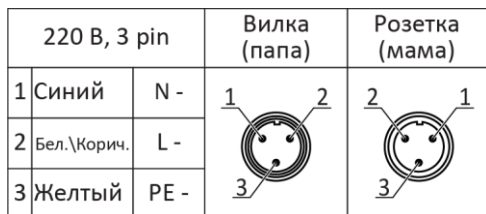
Рисунок 2. Варианты комплектных разъемов.
