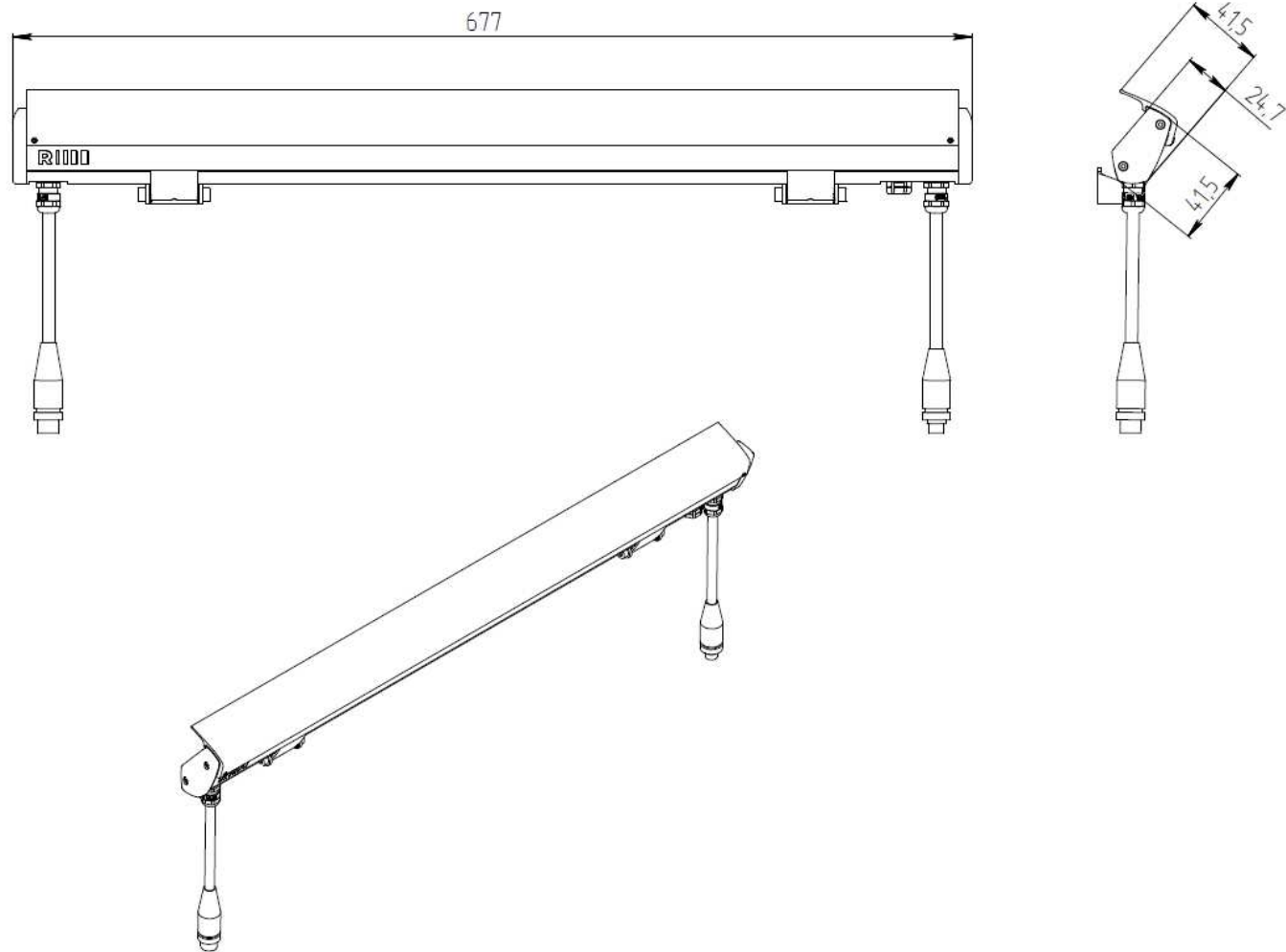
Рисунок 1. Общий вид светильника RAD-L-InS
