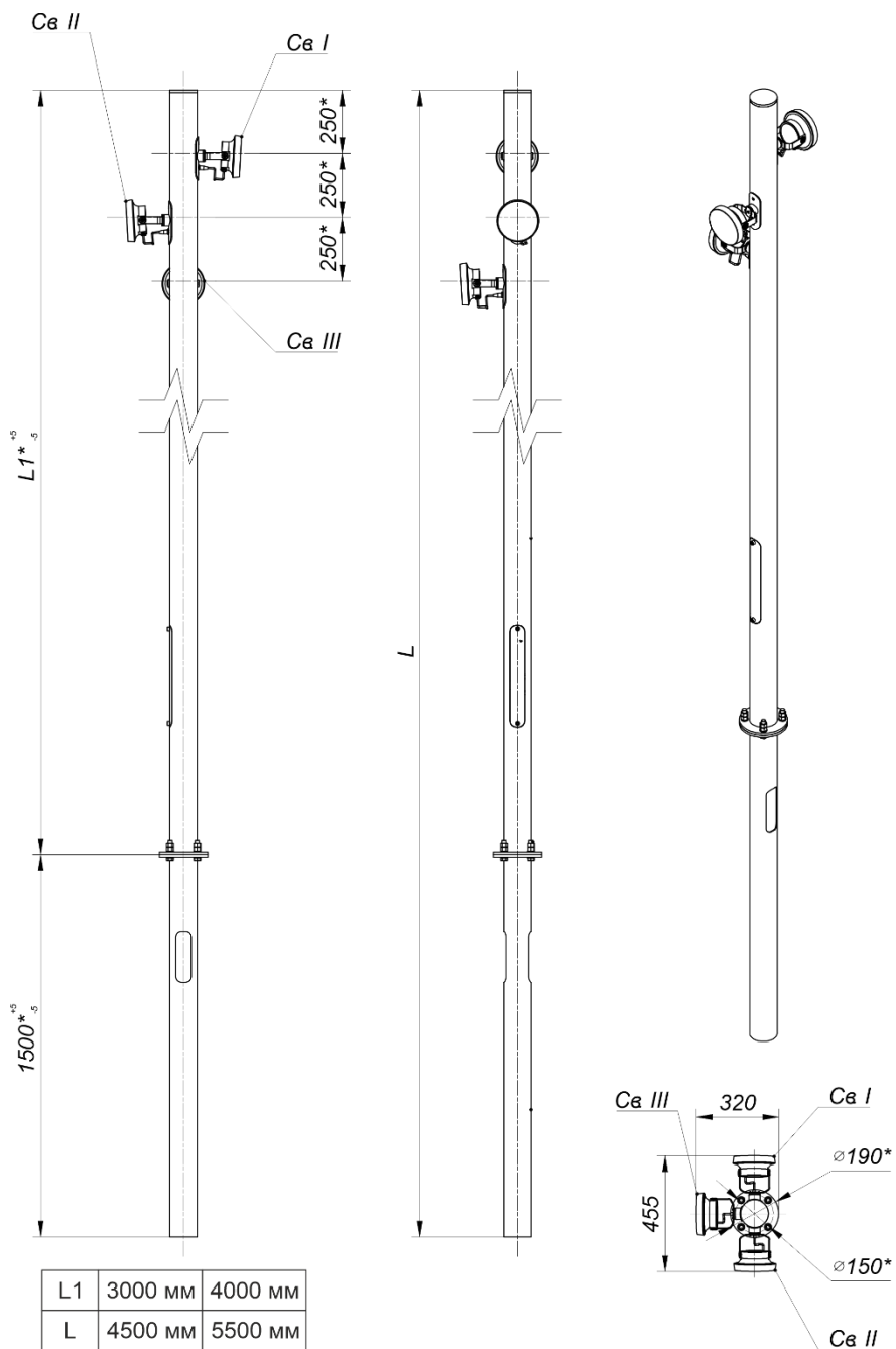
Рисунок 3. Габаритный размеры системы освещения
