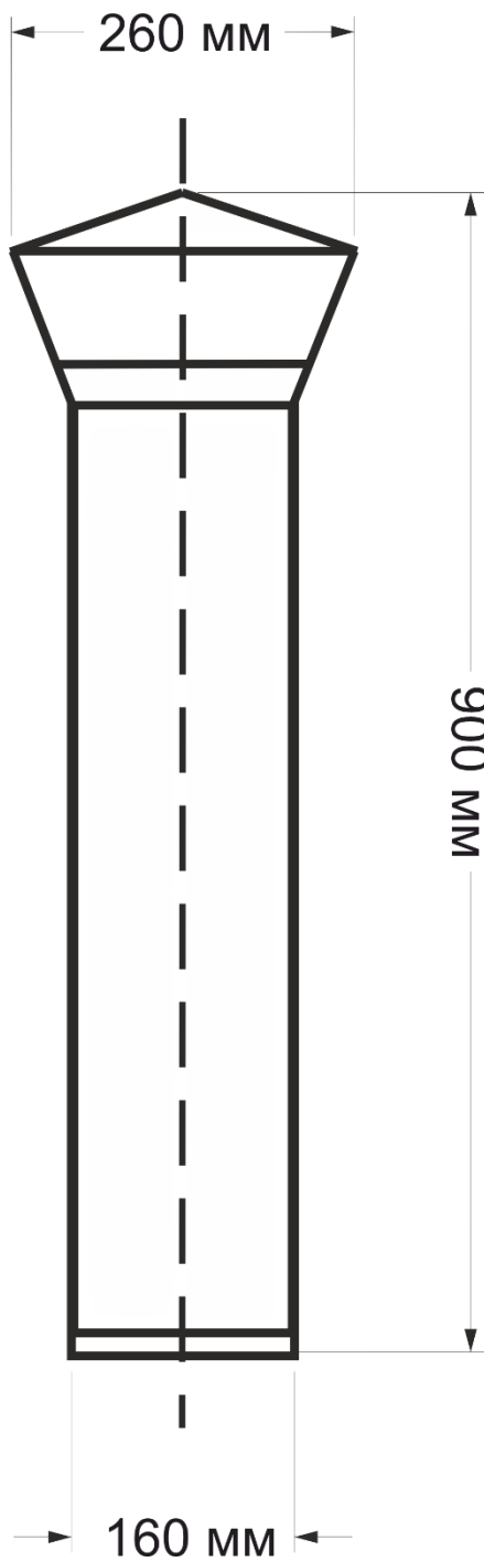
Рисунок 3. Общий вид светильника RAD-STICK
