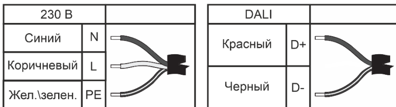
Рисунок 2. Схема подключения питания.
