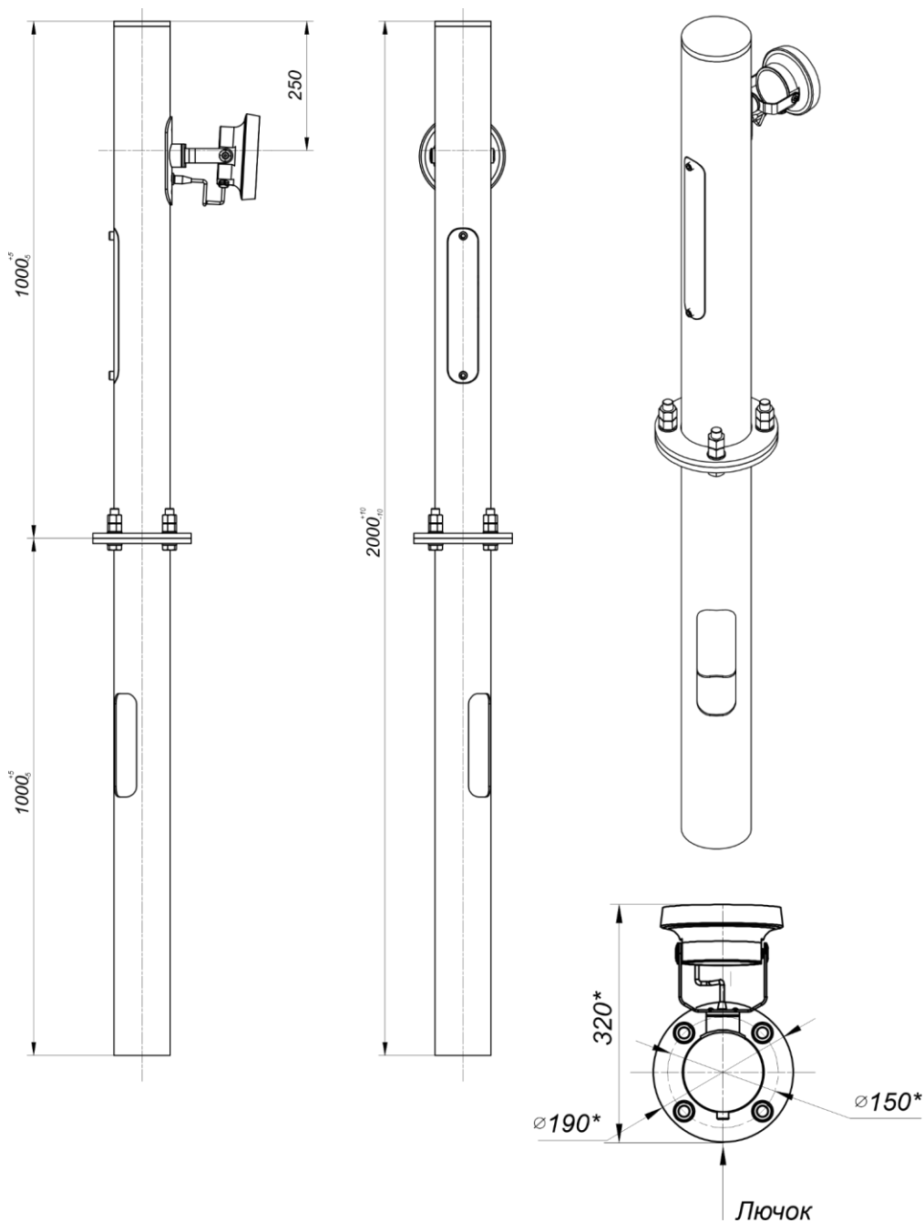
Рисунок 3. Габаритный размеры системы освещения
