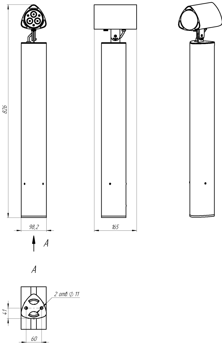
Рисунок 1. Общий вид светильника LOCA SPOT 9
