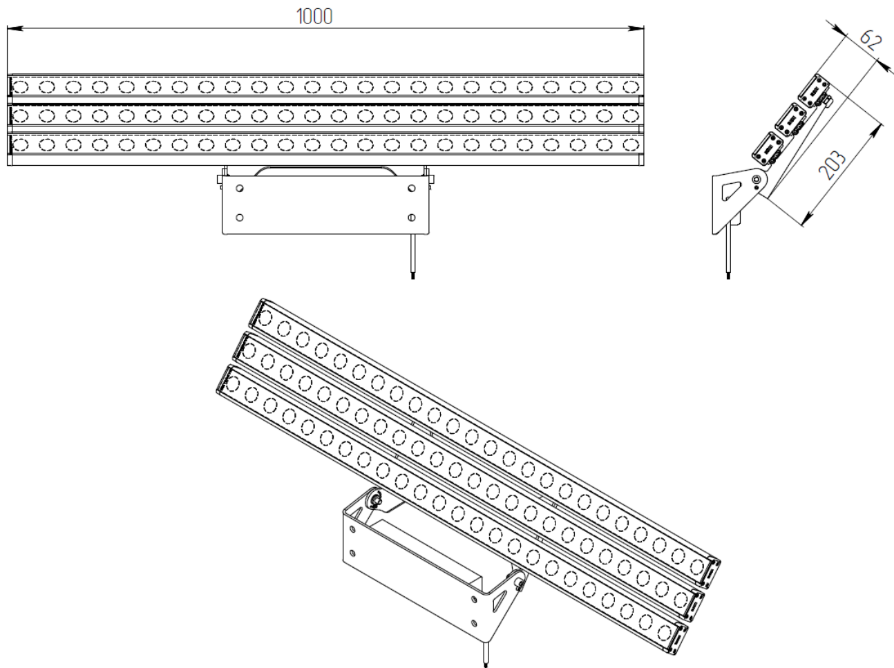
Рисунок 1. Общий вид светильника RAD-L-ST X3
