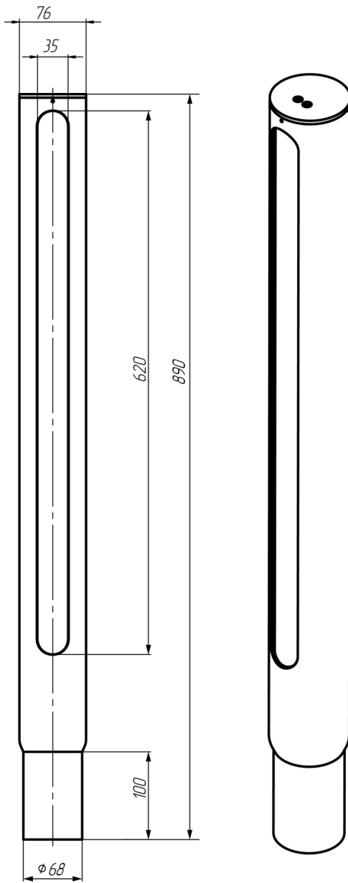
Рисунок 1. Общий вид светильника RAD-STRIP
