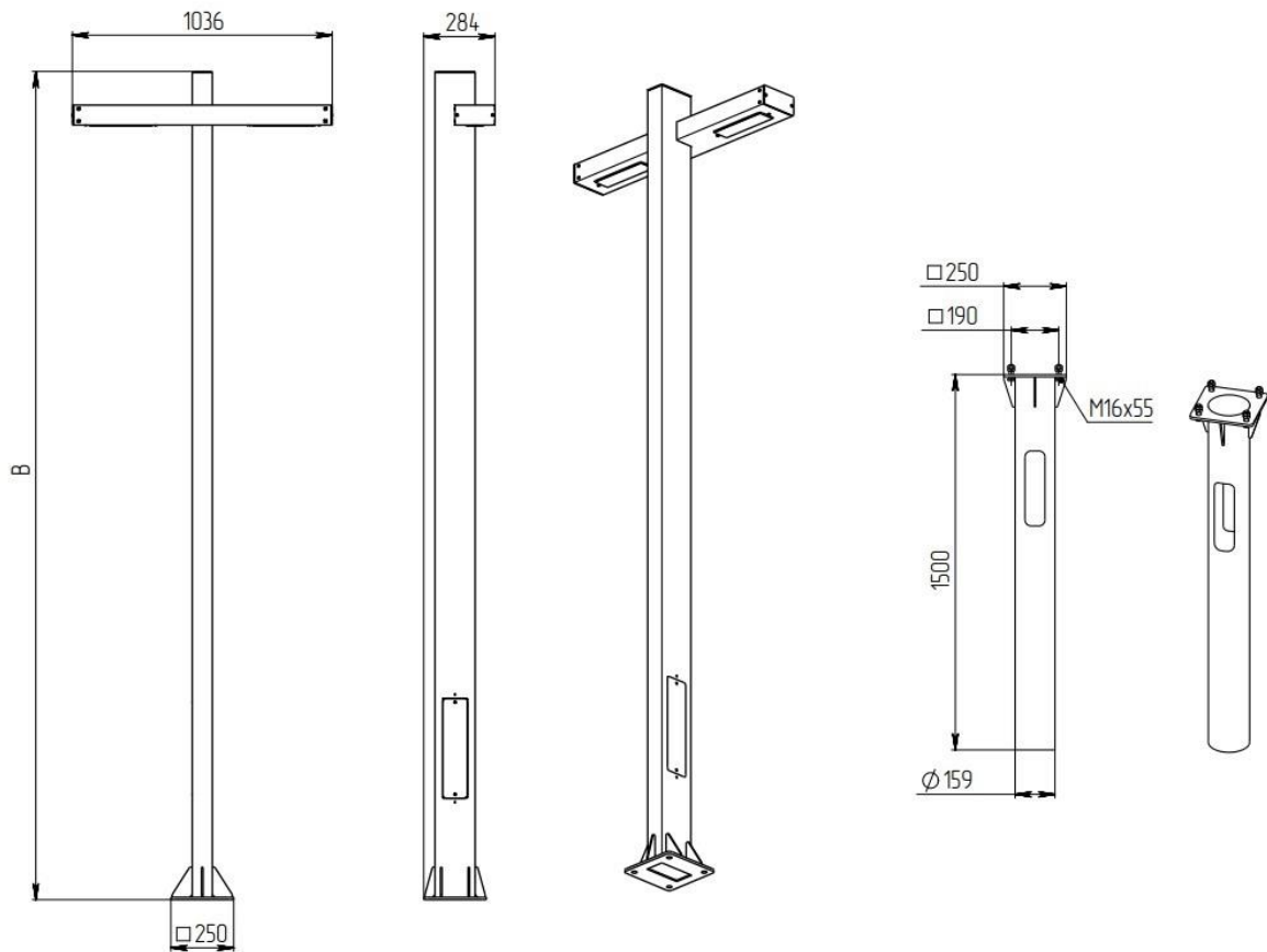
Рисунок 1. Общий вид светильника MALEVICH v2.2
