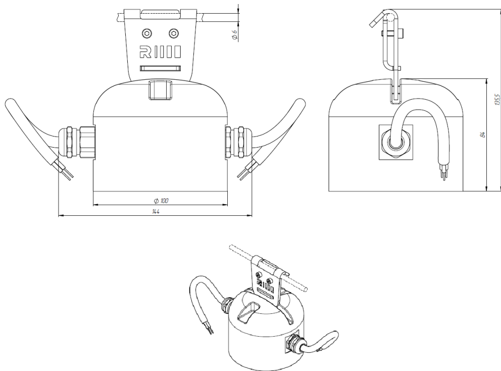
Рисунок 1. Общий вид светильника RAD-SHR
