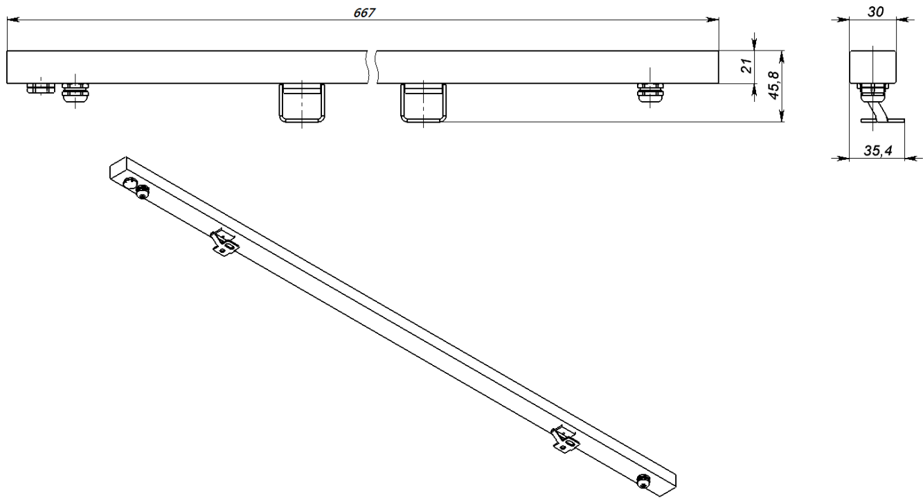
Рисунок 1. Общий вид светильника RAD-L-SL
